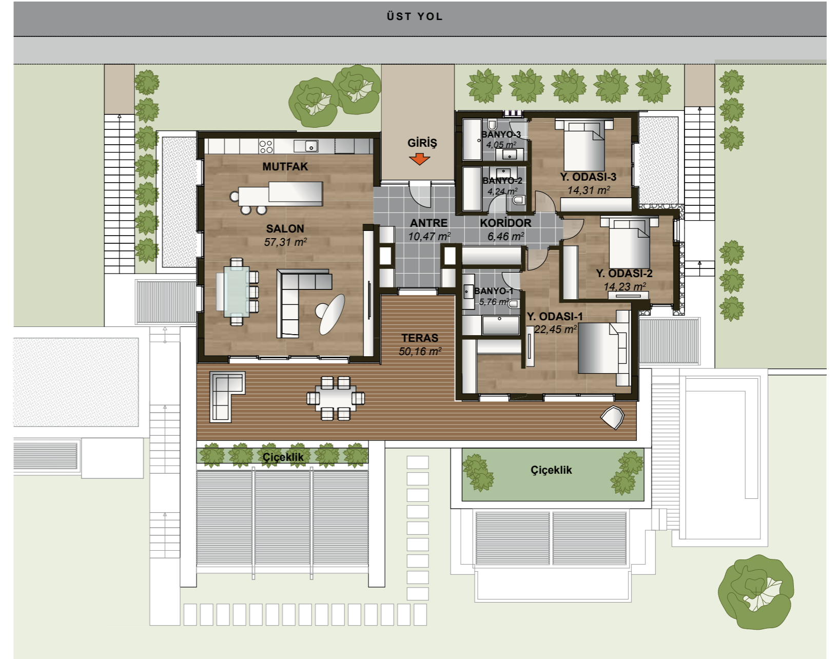
1.Kat Planı
