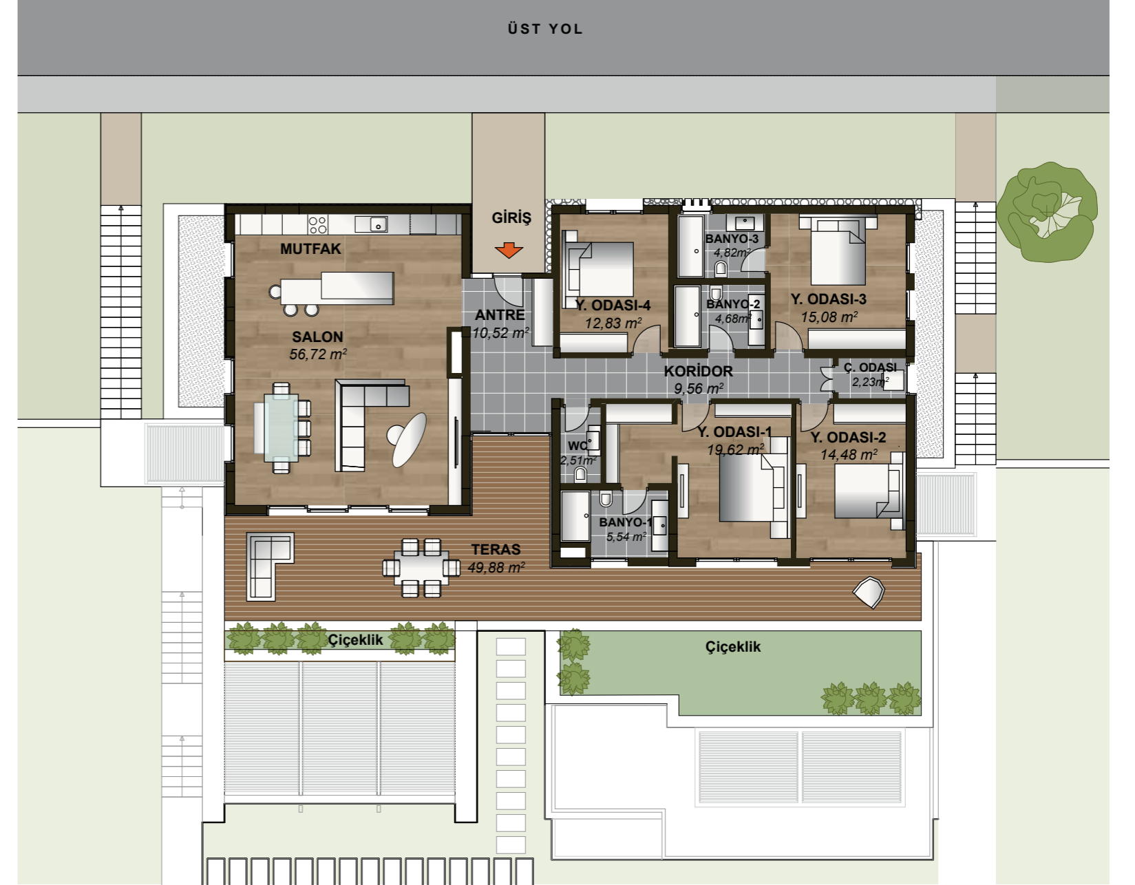
1.Kat Planı
