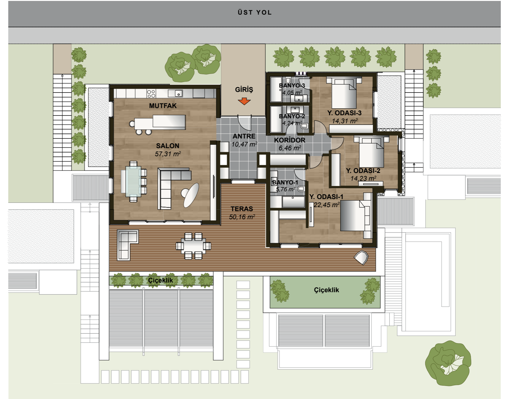
1.Kat Planı
